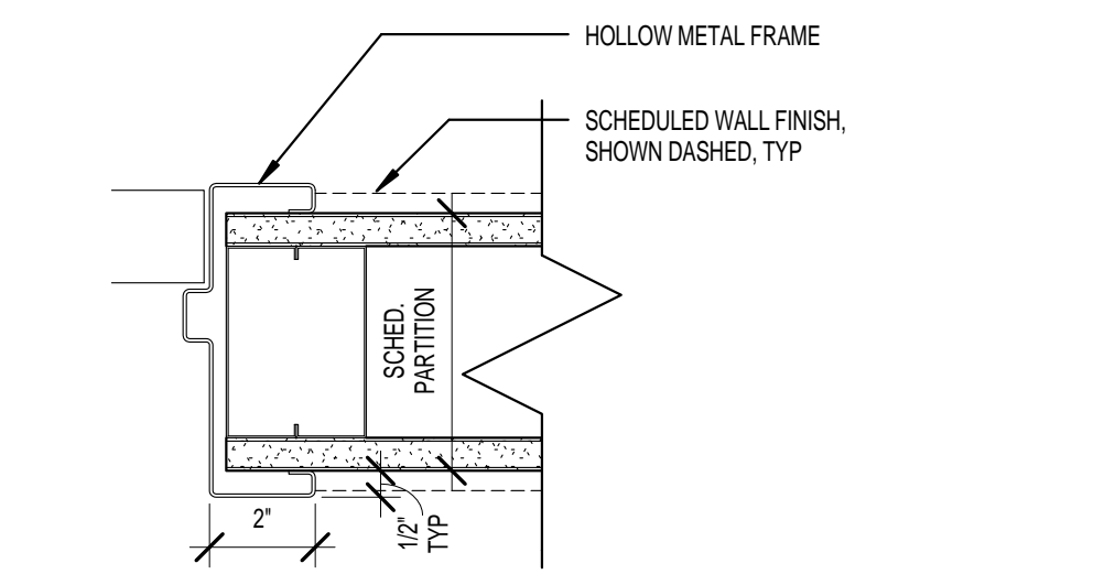
6 DR JAMB DETAIL - TYP GYP BD PARTITION
