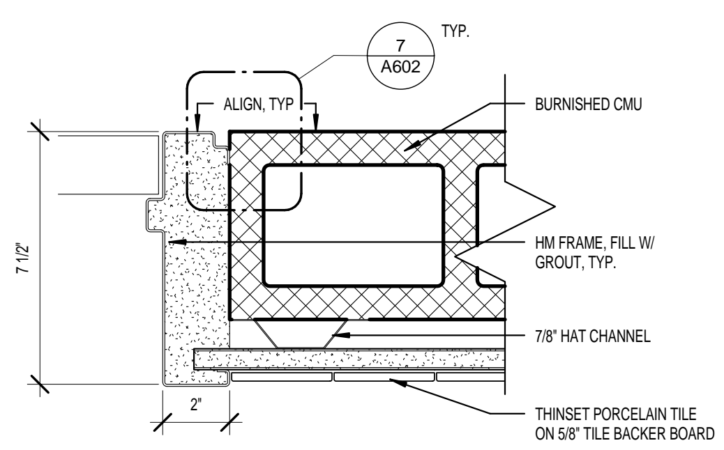
3a DR JAMB DETAIL - CMU - TOILET RM
