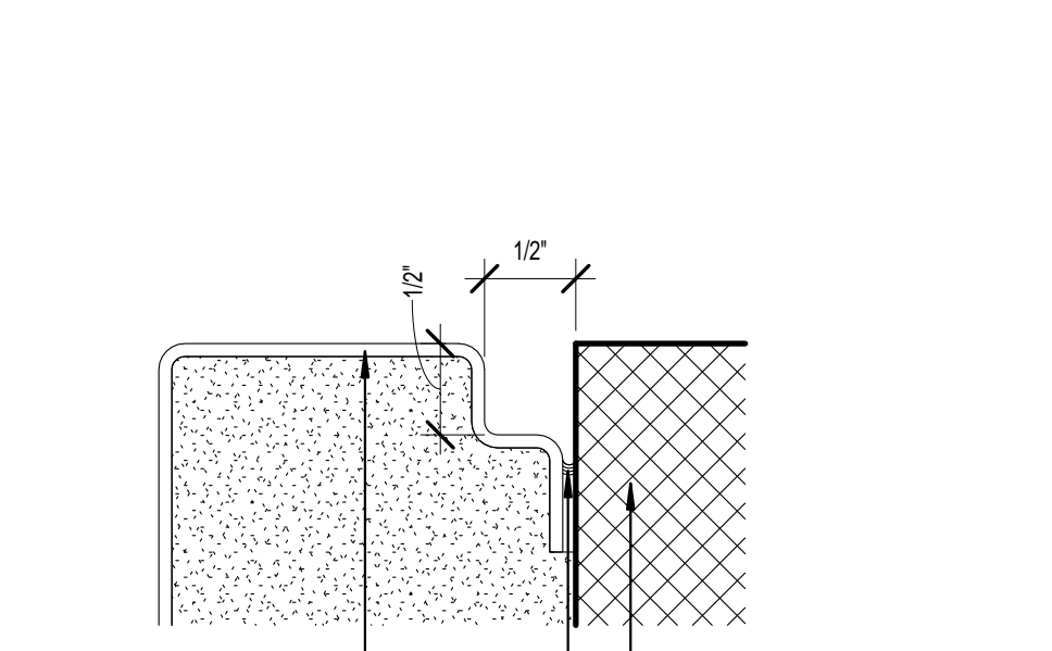
7 DTL @ DOOR JAMB
